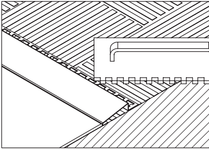
4 Döşemelerin uygulanacağı yerlere mala ile ilave harç sürün.
