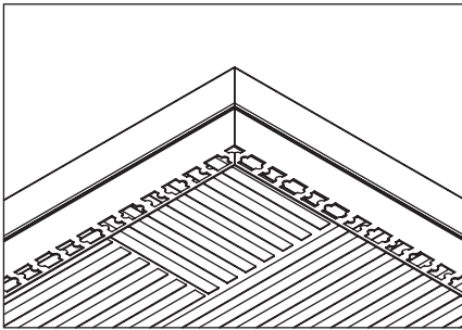
10 45 derece kesim yaptığınız profilleri iç köşelerde birbirine tam olarak oturacak şekilde harca bastırın.
