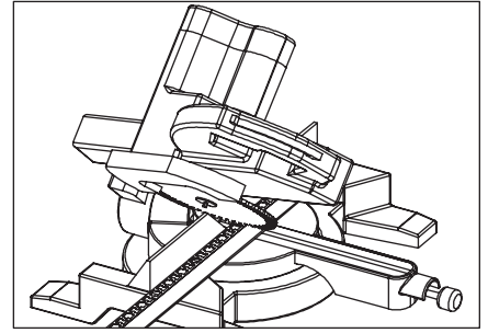
9 İç köşe dönüşlerini sağlamak için her iki profili 45 derece kesin.
