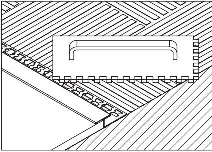
4 Döşemenin uygulanacağı yerlere mala ile ilave harç sürün.
