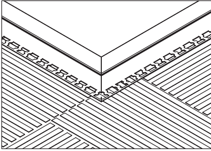
7 45 derece kesim yaptığınız profilleri dış köşelerde birbirine tam olarak oturacak şekilde harca bastırın.
