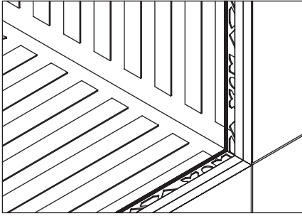
7 45 derece kesim yaptığınız profilleri köşelerde birbirine tam olarak oturacak şekilde harca bastırın.
