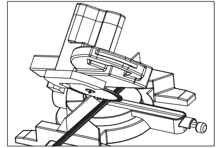
6 Köşe dönüşlerini sağlamak için her iki profili 45 derece kesin.
