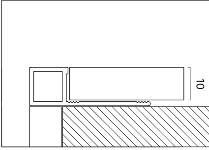
1 Seramiklerin kalınlığına uygun profili seçin.
