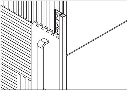
4 Seramiklerin döşeneceği yerlere mala ile ilave harç sürün.
